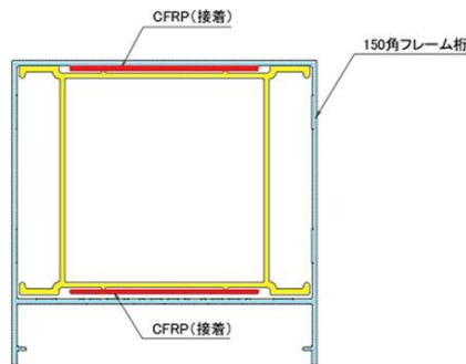
スリーブ補強断面
