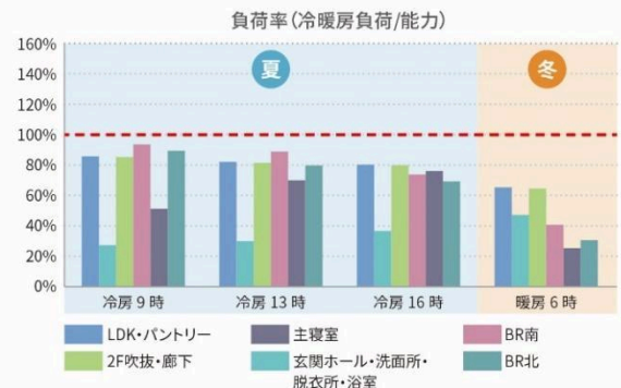
日射遮蔽対策 改善後
