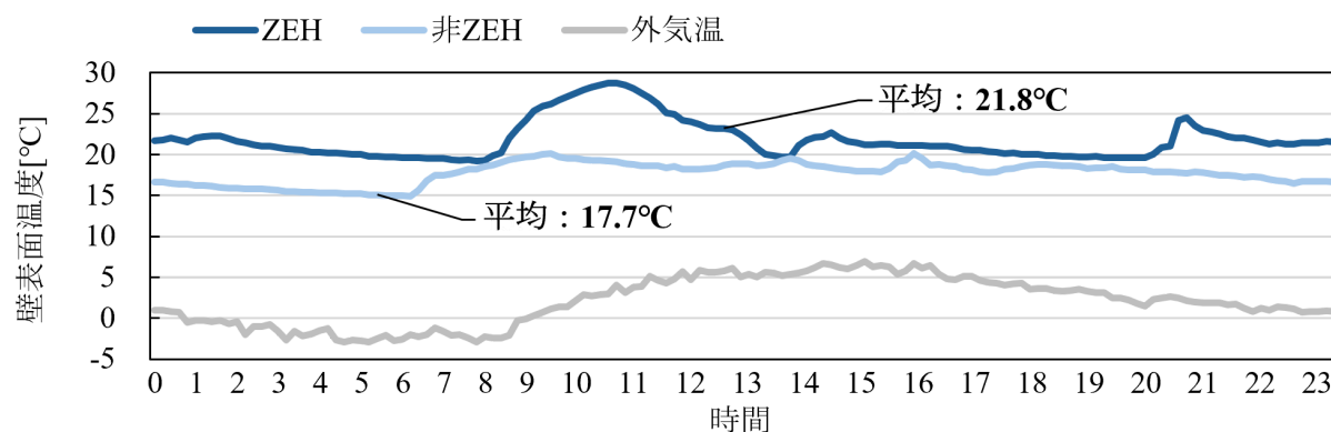
ZEH・非ZEH代表住戸における冬季(2/20)の壁表面温度
