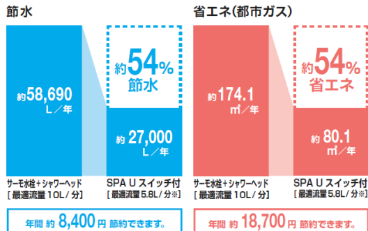
スイッチ付の場合
